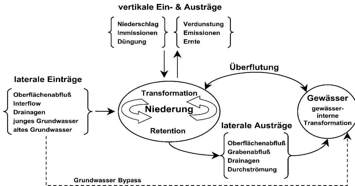
Abbildung 5: Funktionsweise des WETTRANS-Modells (verändert nach TREPEL & KLUGE 2004).
