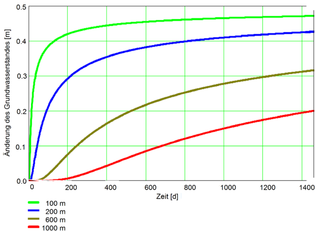
Abbildung 12: Änderung des mittleren Grundwasserstandes in GWL 1 aufgrund der Erhöhung der Torfwasserstände im Polder um 0,5 m in Abhängigkeit vom Abstand zur Polderfläche basierend auf der Sprungantwortfunktion (Busch et al. 1993). Abbildung: A. Wahren.
