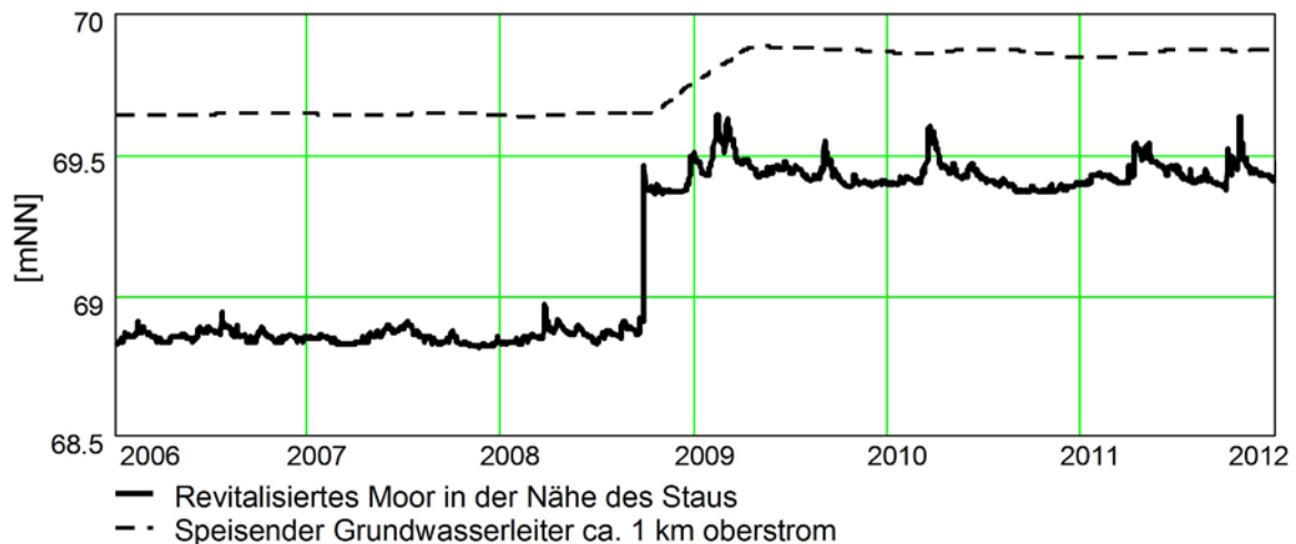
Abbildung 11: Berechneter Grundwasseranstieg nach einer Wiedervernässung (eigene Prinzipskizze basierend auf synthetischen Daten). Abbildung: A. Wahren.
