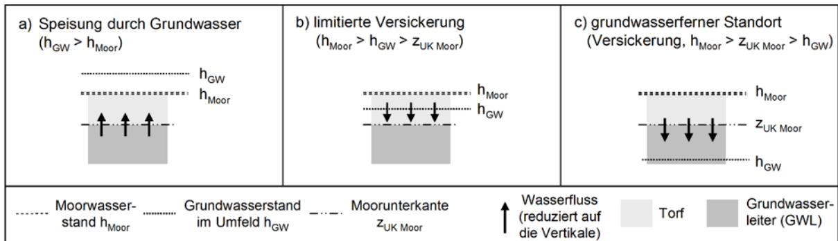
Abbildung 10: Interaktion zwischen Moor und Grundwasser im Umfeld des Moorstandortes. Abbildung: A. Gerner
