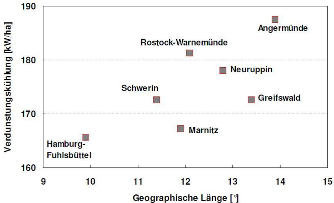
Abbildung 20: Verdunstungskühlung durch Wiedervernässung von Grünland. Es ist die Kühlung dargestellt die sich ergibt, wenn in einem Grünland der mittlere Grundwasserflurabstand von 1 m auf 0–0,1 m erhöht wird.
