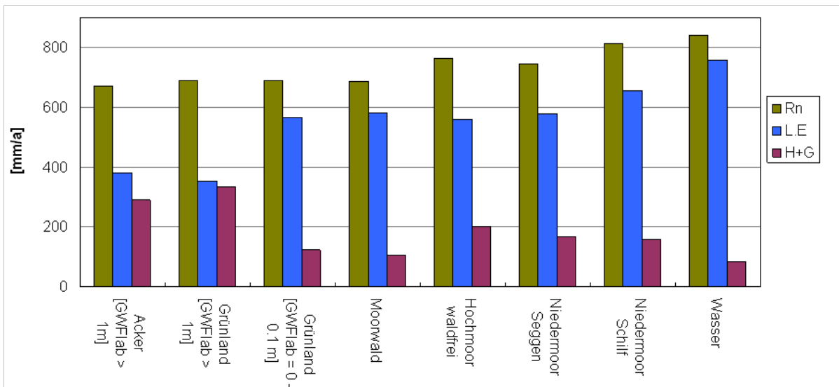
Abbildung 16: Vegetationsabhängige Komponenten der Energiebilanz (L.E nach ROMANOV mit AKWA-M® berechnet, H+G als Restglied). Abbildung: K. Brust.
