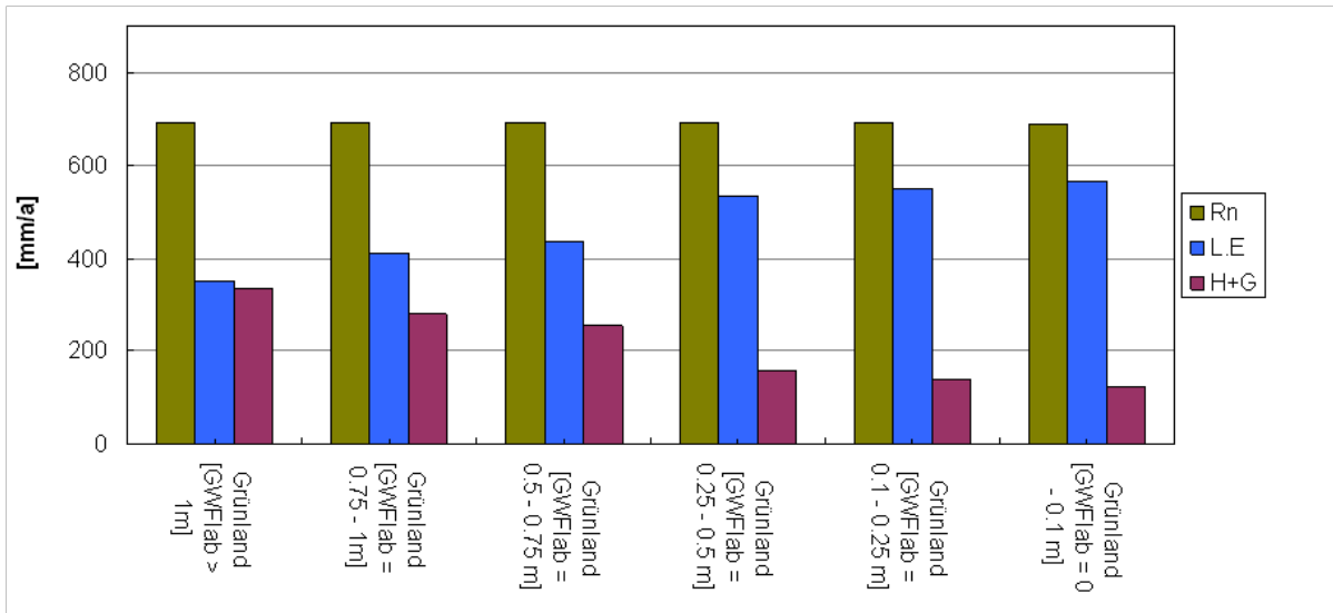
Abbildung 15: Komponenten der Energiebilanz (L.E nach Romanov mit AKWA-M® berechnet, H+G als Restglied) über Grünland mit unterschiedlichen Entwässerungstiefen. Abbildung: K. Brust.
