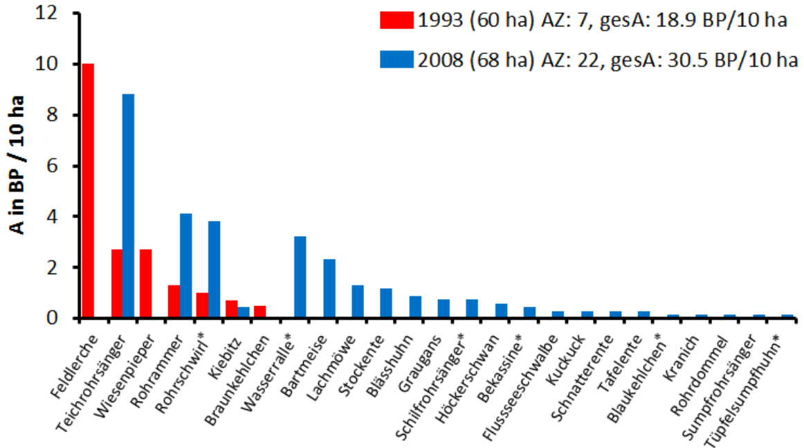
Abbildung 18: Abundanzen der Brutvögel vor und acht Jahre nach der Wiedervernässung im Polder Randow-Rustow, Mecklenburg-Vorpommern (aus HEROLD 2012). * = Leitart der Flusstalmoore, A = Abundanz, BP = Brutpaare, AZ = Artenzahl, gesA = Gesamtabundanz.
