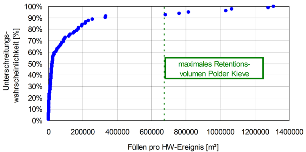
Abbildung 8: Empirische Unterschreitungswahrscheinlichkeit der Hochwasserfüllen der Elde am Pegel Wredenhagen (1983-2011). Abbildung: A. Wahren.
