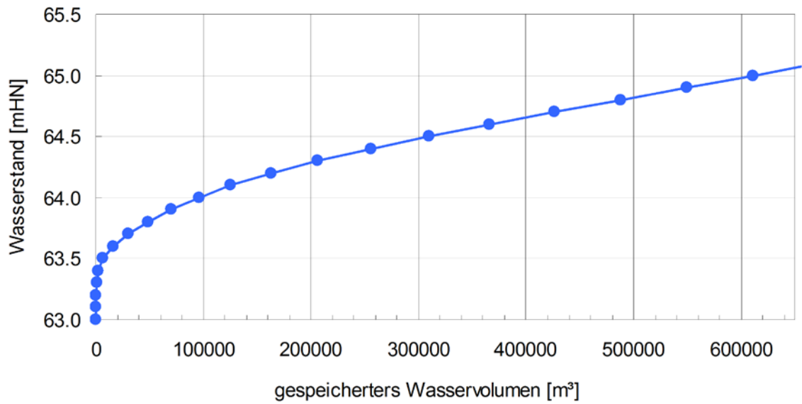
Abbildung 7: Speicherinhaltslinie für den Polder Kieve (Beziehung zwischen Wasserstand und gespeichertem Wasservolumen) generiert aus DGM (© GeoBasis-DE/M-V 2013). Abbildung: A. Wahren.
