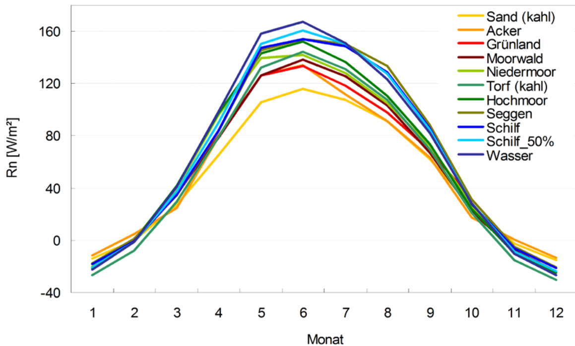
Abbildung 14: Strahlungsbilanzen im Jahresgang für verschiedene Landnutzungen. Abbildung K. Brust.
